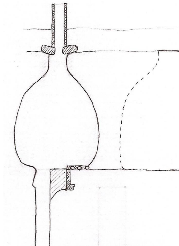
Sección del Silo G. En su parte central tiene unos 230 cm de anchura y de altura unos 330 cm (Dibujo propio a partir de BERTRAND, SÁNCHEZ, 2008)
